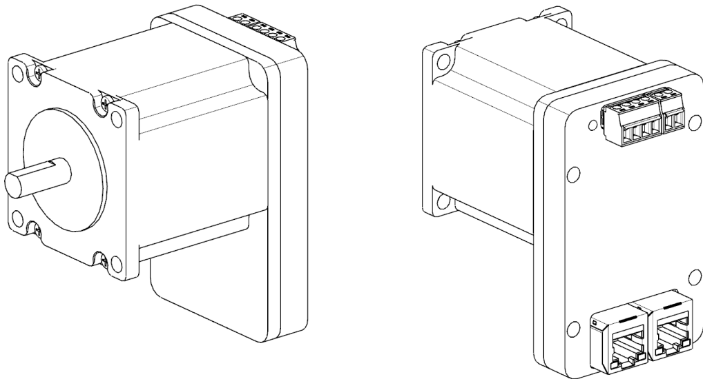
产品外形图
