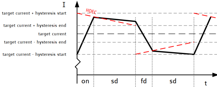
on 为绕组充电段 sd 为慢衰减段 fd 为快衰减段
