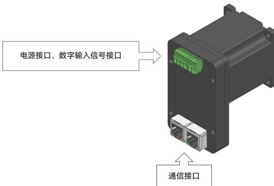
接口示意图
