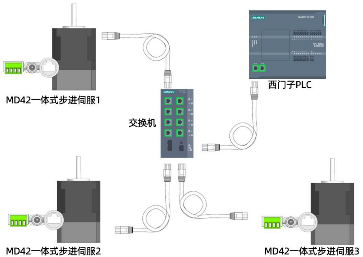
星型网络拓扑
