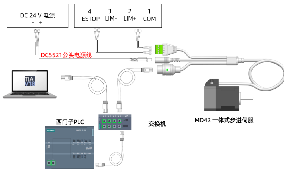
系统连接
