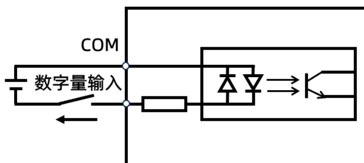
NPN接线
