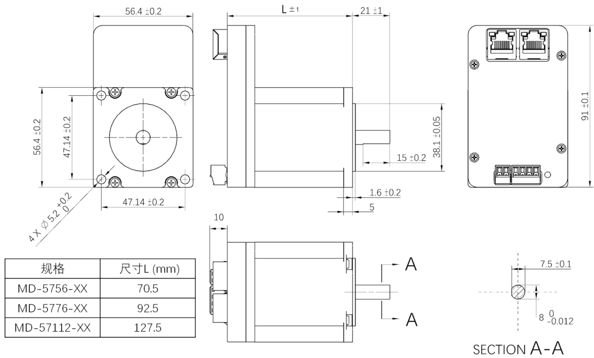
产品尺寸图
