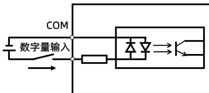
PNP接线
