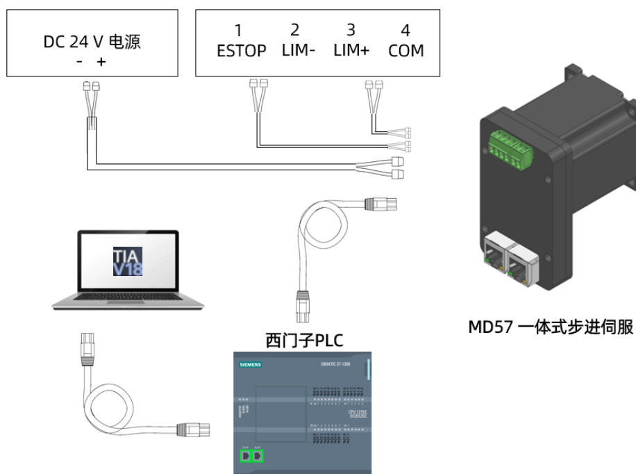
系统连接
