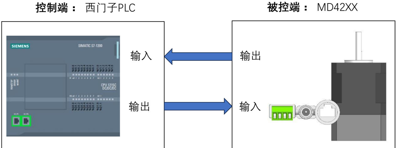
控制端与被控端示意图
