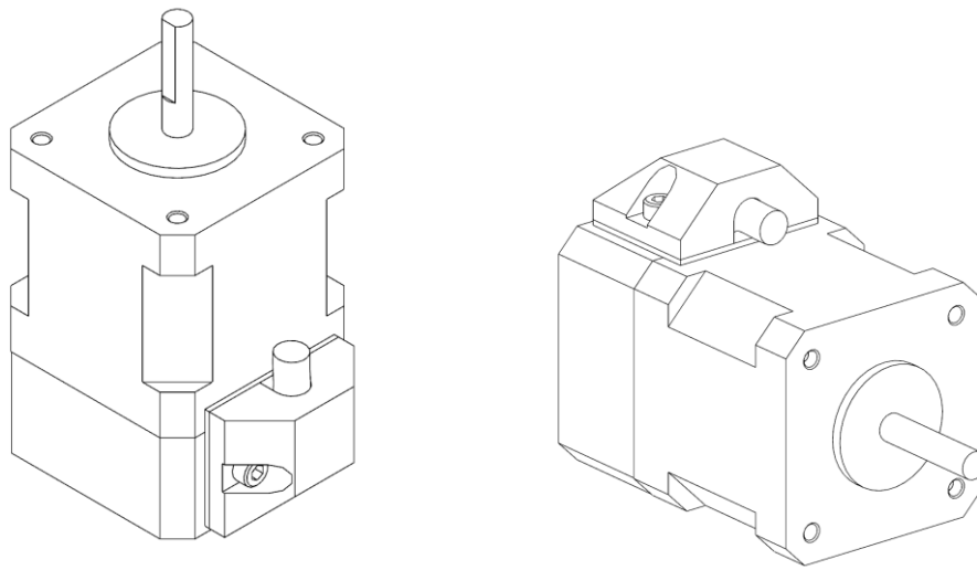
产品外形图
